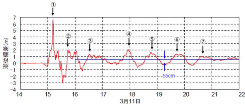
圖一 岩手南部沖GPS波浪計で捉えた津波の初期の波形
