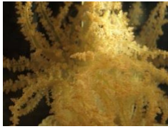
海蜂海葵(学名: Phyllodiscus semoni Kwietniewski)
