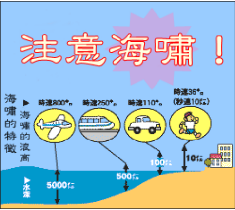
海啸的传播速度与水深关系
