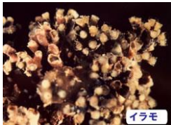
Iramo 水母（水母的一种；学名: Stephanoscyphus racemosum ）
